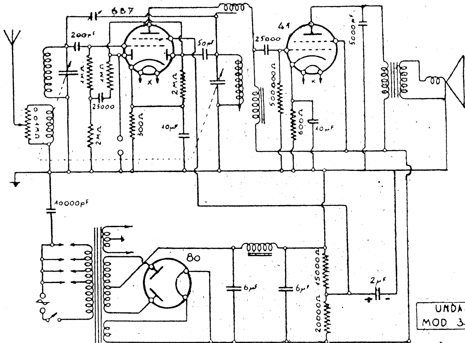
UNDA RADIO. — Mod. « 337 ». — Produzione 1936. — Media frequenza: 450 kHz.
